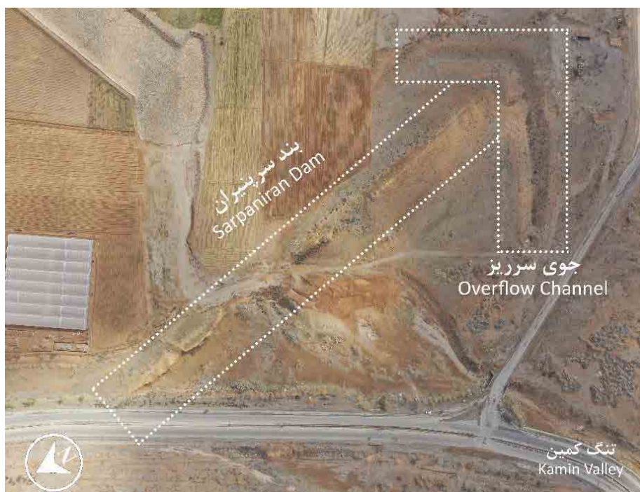
شکل ۱۶. دید هوایی سد سرپنیران و جوی سرریز آب در انتهای جنوبی سد (نگارندگان، ۱۳۹۹).
