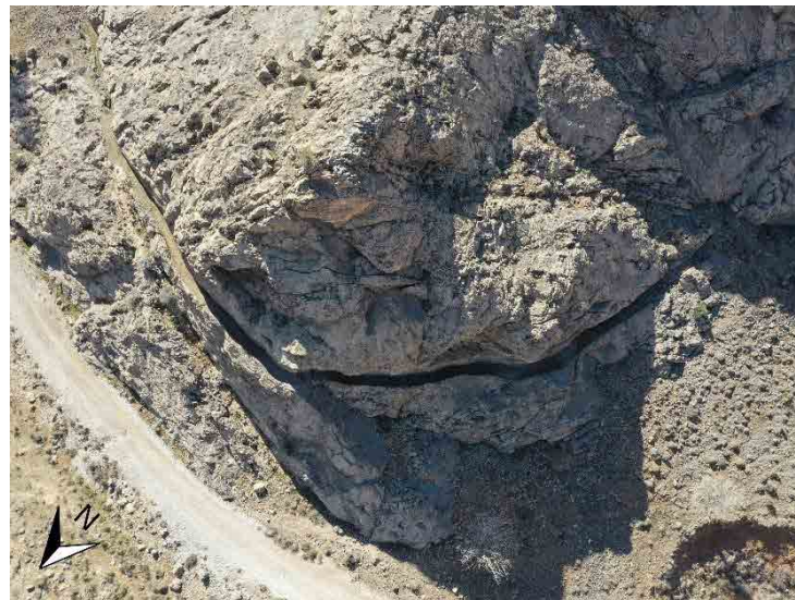
شکل ۲۶. دید هوایی از آبراه دست‌کند کرانه خاوری در دهانه تنگ بلاغی (نگارندگان، ۱۳۹۹). Fig. 26. Aerial view of the east bank's steep waterway in the mouth of Tangbolaghi (Authors, 2019).
