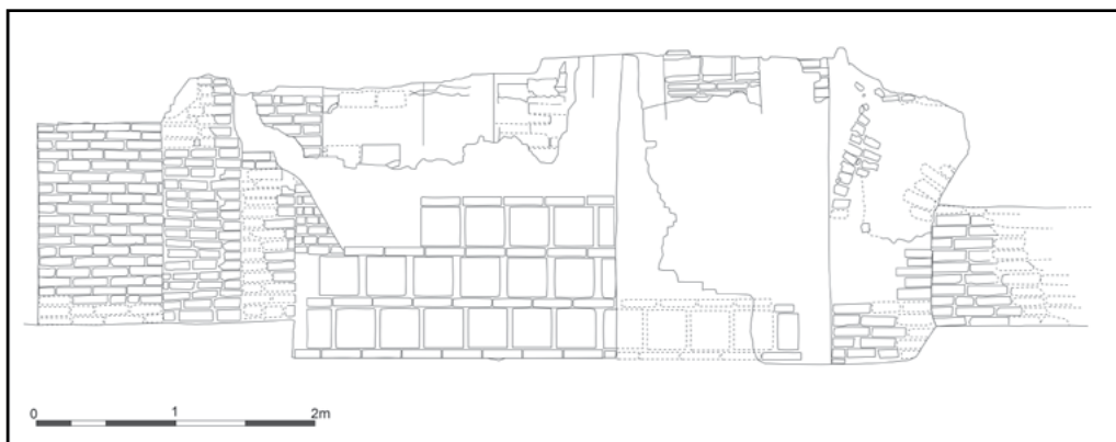
تصویر ۱۲: برش A-A کوره آجرپزی/آهک‌پزی شماره ۱ (ترسیم از: حامد رضایی، ۱۳۸۱). Fig. 12: Section A-A of lime and brick-manufacturing kiln no. 1 (Drawing by: Hamed Rezaei, 2002).
