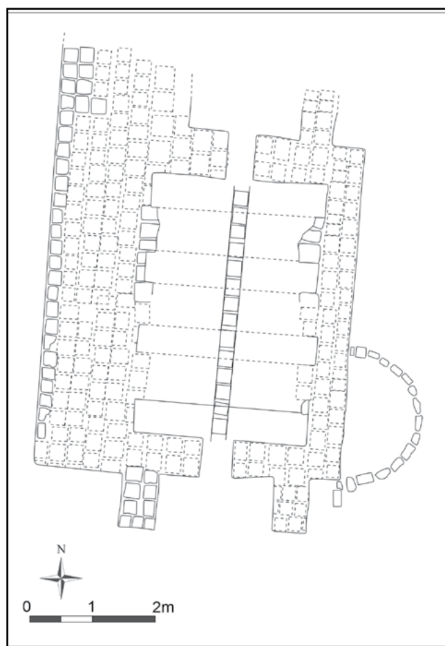
تصویر ۸: نقشه کوره آجرپزی شماره ۱ (ترسیم از: حامد رضایی، ۱۳۸۱). Fig. 8: Plan of brick-manufacturing kiln no. 1 (Drawing by: Hamed Rezaei, 2002).
