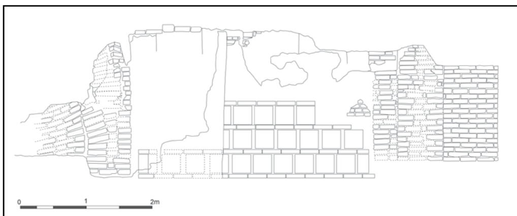
تصویر ۱۳: برش B-B کوره آجرپزی/آهک‌پزی شماره ۱ (ترسیم از: حامد رضایی، ۱۳۸۱). Fig. 13: Section B-B of lime and brick-manufacturing kiln no. 1 (Drawing by: Hamed Rezaei, 2002).
