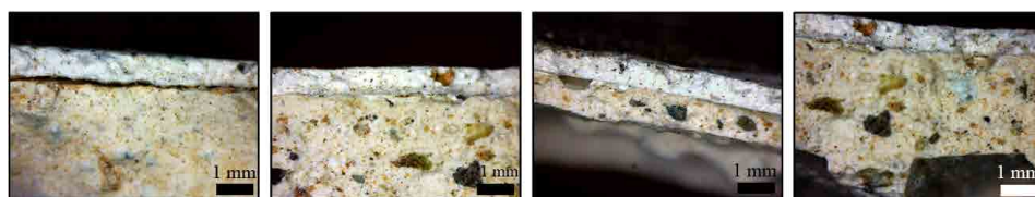
تصویر ۲۳. تصاویری از مقطع لایه آستر و بستر با کمک میکروسکوپ دیجیتالی، تفاوت رنگ و بافت و تخلخل در دو لایه آستر و بستر (نگارندگان، ۱۴۰۰).
