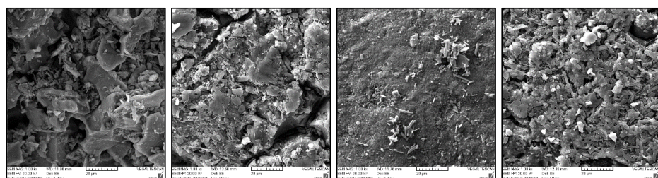
تصویر ۲۶. تصاویر تهیه شده از رنگ قرمز (2021.Q.IH.6)، پرکننده لایه تدارکاتی (2021.Q.IH.7)، قهوه‌ای براق (2021.Q.IH.8) و قلم‌گیری (2021.Q.IH.9) با بزرگ‌نمایی ۱۰۰۰ برابر (از سمت راست)، (نگارندگان، ۱۴۰۰).
