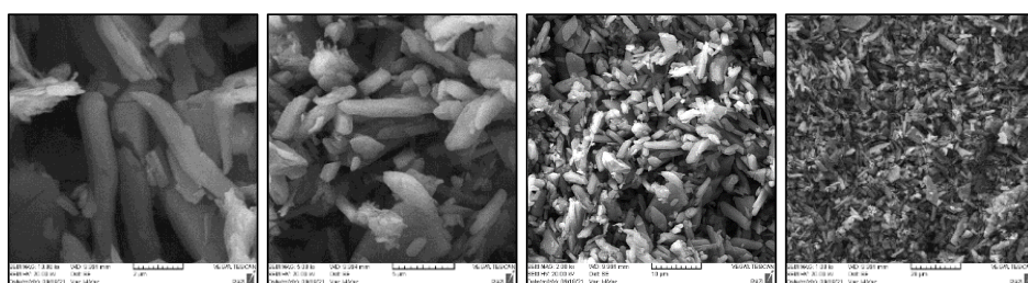
تصویر ۲۴. تصاویر تهیه شده از لایه چینی (2021.Q.IH.1) با بزرگ‌نمایی ۱۰۰۰، ۲۰۰۰، ۵۰۰۰ و ۱۰۰۰۰ برابر (نگارندگان، ۱۴۰۰).
