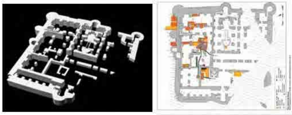
تصویر ۸. نقش و طرح ایزومتریک بنای بازیان (Déroche, 2015: 11).
