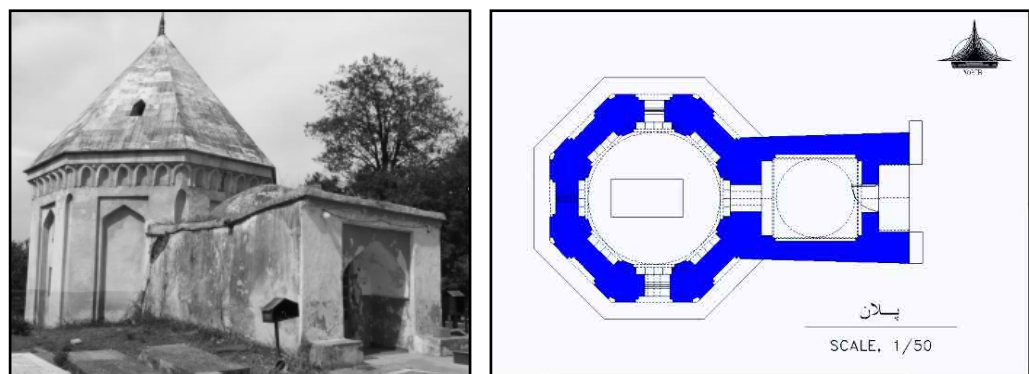
نقشه ۲: نقشه و نمای مسجد برج مقبره‌ای سیدعلی کیاسلطان (نگارندگان، ۱۳۹۹).
