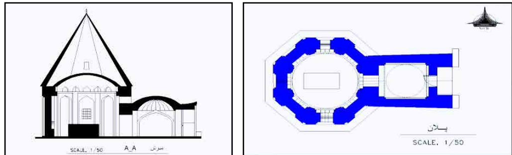
نقشه ۱: نقشه و برش نمای برج مقبره‌ای سیدعلی کیاسلطان (نگارندگان، ۱۳۹۹).
