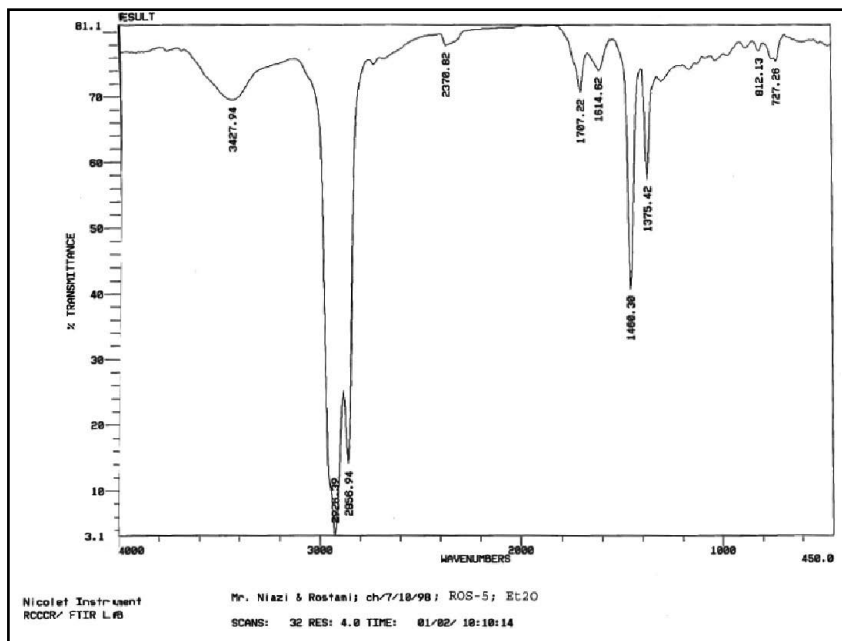
تصویر ۱۱. طیف FT-IR نمونه الوار چوبی طولی از قسمت درون کشتی که با حلال دی‌اتیل اتر استخراج شده است (مرکز آنالیز FT-IR پژوهشکده حفاظت و مرمت).
