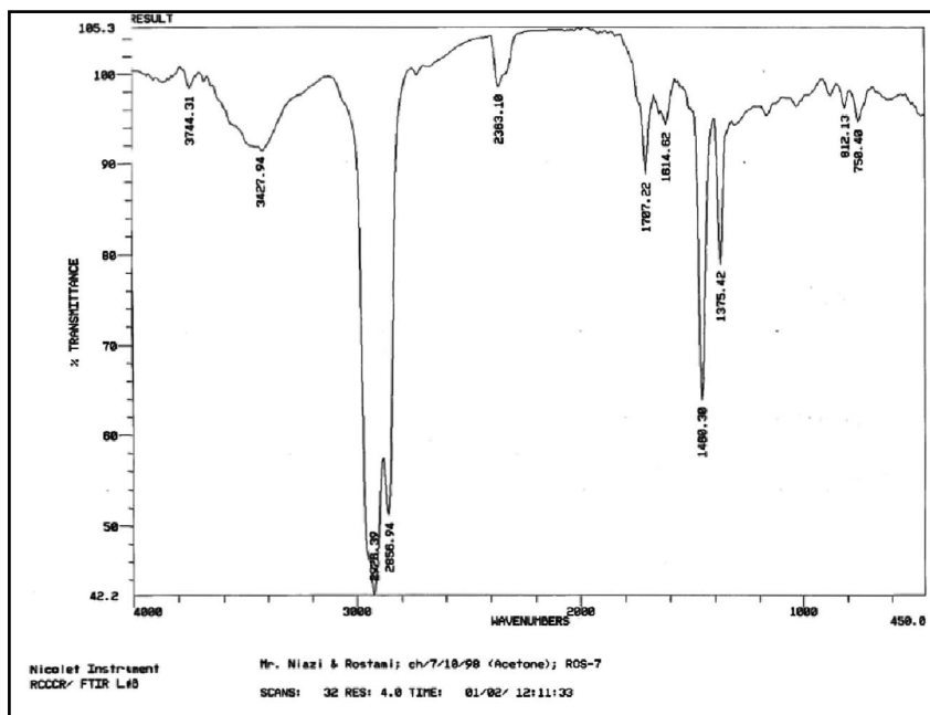
تصویر ۱۲. طیف FT-IR نمونه الوار چوبی طولی از قسمت درون کشتی که با حلال استن استخراج شده است (مرکز آنالیز FT-IR پژوهشکده حفاظت و مرمت).
