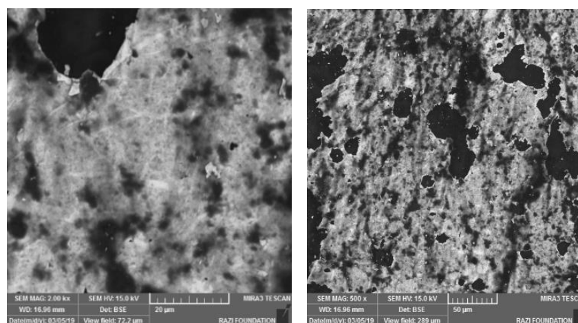
تصویر ۱۷. تصاویر میکروسکوپ الکترونی از ورق طلای نقاشی مورد مطالعه (نگارندگان، ۱۴۰۰). Fig. 17. SEM-BSE images of the gold leaf in the studied painting (Authors, 2022).
