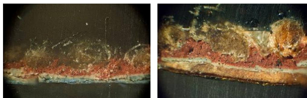
تصویر ۱۶. لایه‌های تشکیل دهنده نقاشی در قسمت طلایی (راست) و زمینه آبی (چپ) (نگارندگان، ۱۴۰۰). Fig. 16. The layers of the painting in the gilded part (right) and the blue background (left) (Authors, 2022).
