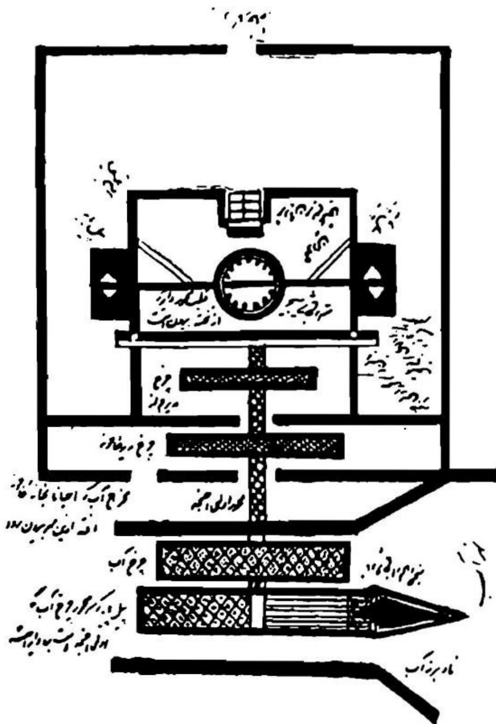
تصویر ۷. آسیای روغن حافظ اصفهانی، قرن نهم هجری قمری (محبوبی، ۱۳۸۳: ۲۲۲).
