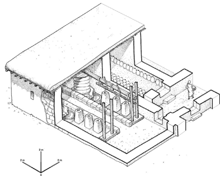
تصویر ۲. عصاره با شیوهٔ اهرم و وزنه، شحیم لبنان، قرن ۵ و ۶ م. (Waliszewski, 2014: fig.43). Fig. 2. Lever and weight press at Chehime, Lebanon (Waliszewski, 2014: fig. 43).
