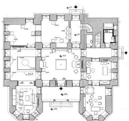
تصویر ۱۵. نمای جنوبی و نقشه طبقه همکف «کوکب احمدشاهی» نیاوران (دفتر فنی کاخ نیاوران).
