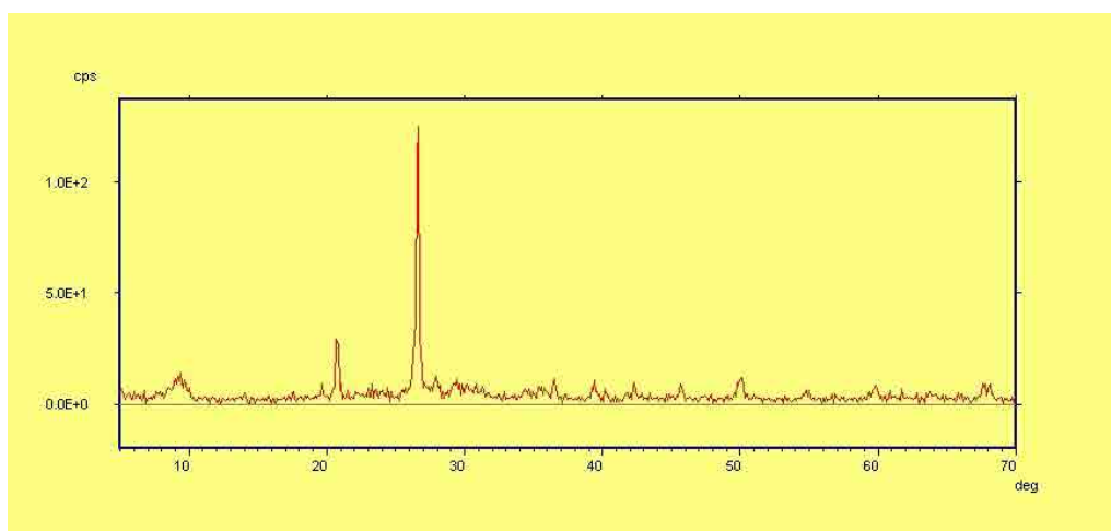
تصویر ۷-۹. طیف XRD نمونه شماره ۹ (H.N.L.1)، نگارندگان، (۱۳۹۸).
