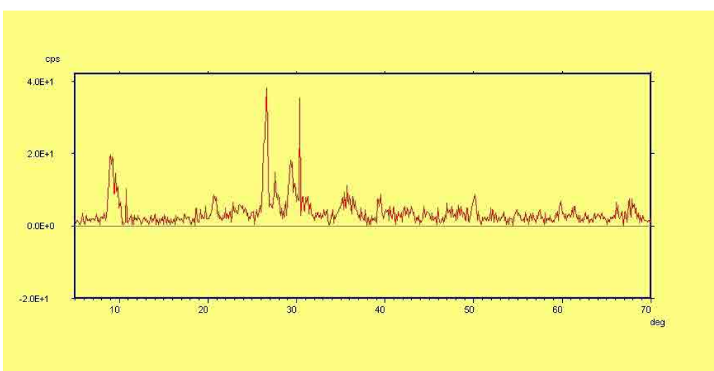
تصویر ۷-۴. طیف XRD نمونه شماره ۴ (L.H.A.S)، نگارندگان، (۱۳۹۸).
