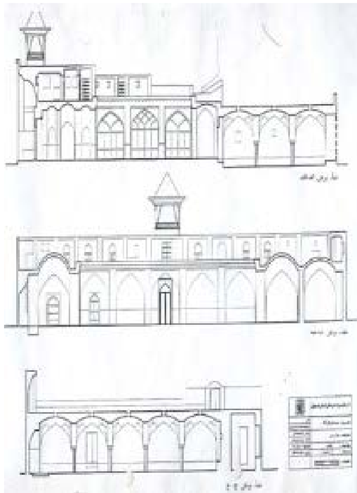
نقشه ۲. برش نمای بیرونی مسجد علیقلی آقا (مرکز اسناد میراث فرهنگی اصفهان، ۱۳۷۸).
