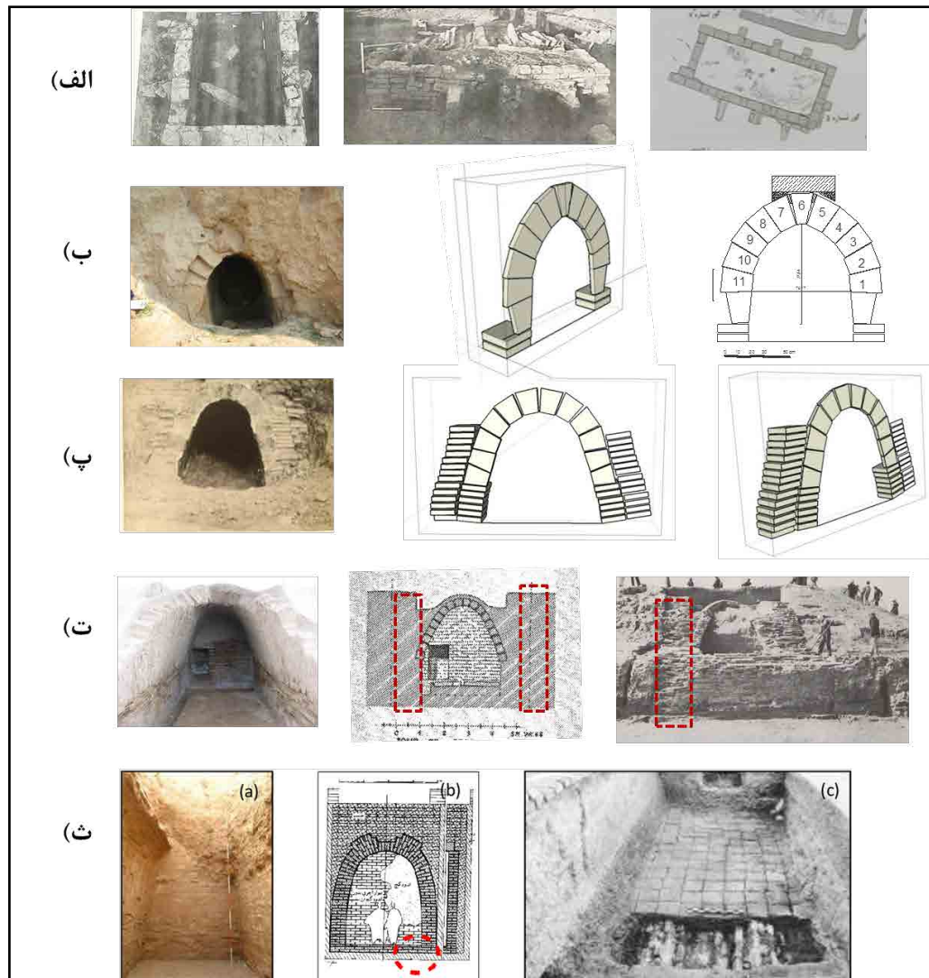
شکل ۵: پنج شیوه از تمهیدات پایداری در طاق‌های آهنک در دوره ایلام: الف) چگاسفلی: ایجاد پشتبندهای عمود بر دیواره طاق (مقدم، ۱۳۹۴: ۱۰۵ و ۷۱). ب) شوش: قرار دادن یک آجر بر روی رأس طاق (نگارنده، ۱۴۰۳). پ) شوش: پرکردن پشت طاق از شروع تا شانه (Dumckenom, 1931). ت) هفت‌تپه: ایجاد دیوار ضخیم و مرتفع در پشت طاق (نگارنده، ۱۴۰۲؛ نگهبان، ۱۳۷۲، ۱۰۴ و ۷۷). ث) چغازنبیل: ایجاد ضخامت در بخش ایوارگاه طاق (نگارنده، ۱۴۰۳؛ گیرشمن، ۱۳۷۵: ۹۸ و ۲۵۹).
