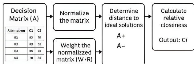
شکل ۵. مراحل اجرای مدل تصمیم‌گیری چند معیاره TOPSIS در ارزیابی روایت فرهنگی (یافته‌های پژوهش)
