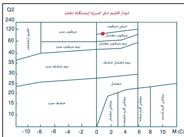
شکل ۱۱. نمودار اقلیم نمای آمبرژه ایستگاه تکاب (قدری، ۱۳۸۸: ۶۲)
