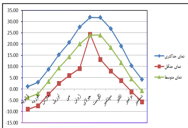
شکل ۶. نمودار نوسانات متوسط، حداقل و حداکثر دمای ماهانه دوره آماری ۳۳ ساله ۱۹۹۰-۲۰۲۳ (برحسب درجه سانتی‌گراد)
