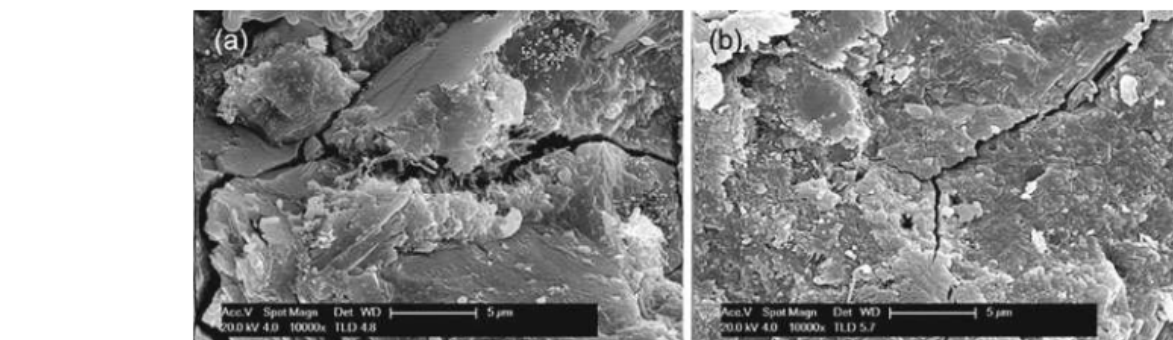
شکل ۶ تصویر SEM از نمونه تحت درمان سمت چپ: اعمال در مرحله ابتدایی و سمت راست: درمان با اکسید گرافن پس از ۲۸ روز از گیرش (Faria et al., 2017)
