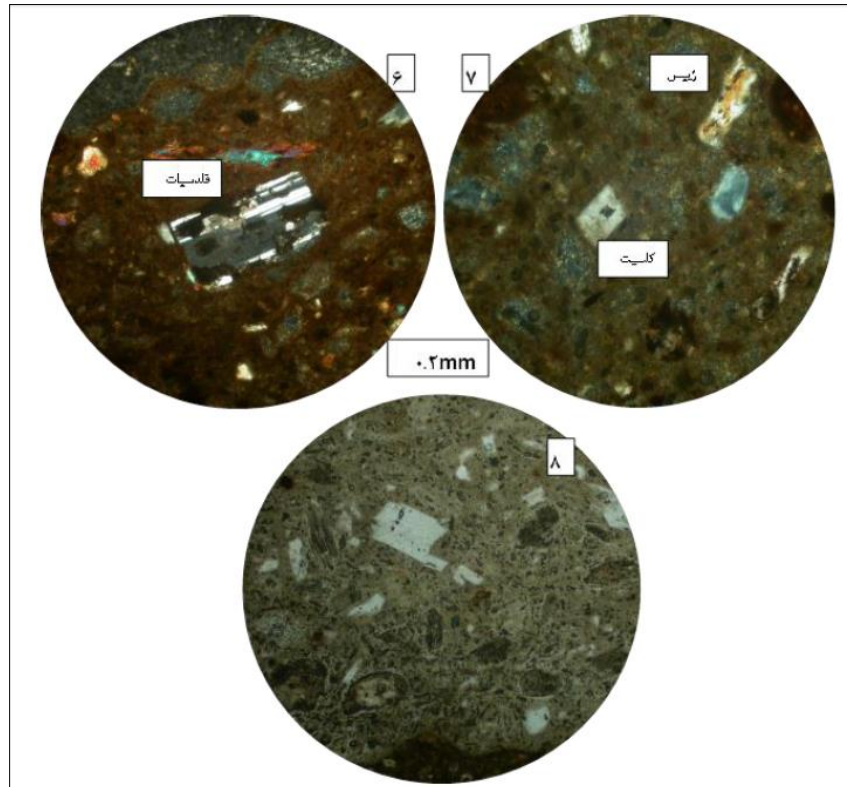
شکل ۷. راست: کانی‌های فیلوسیلیکاته و ژئوپس در لایه آستر؛ چپ و مرکز: کانی‌های فلدسپار و کلسیت به فرم درشت بلور موجود در لایه بستر
