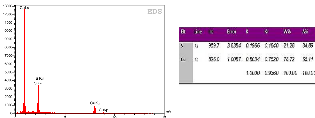
شکل ۱۳. طیف و نتایج EDX از فاز C
