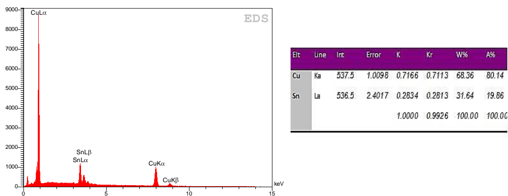
شکل ۱۲. طیف و نتایج EDX از فاز B
