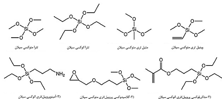
شکل ۳. ساختار مولکولی تعدادی از آلکوکسی سیلان های پر کاربرد مانند تترااتوکسی سیلان، تترااتوکسی سیلان، متیل تری متوکسی سیلان و... (Kudryavtsev & Figovsky, 2015)
