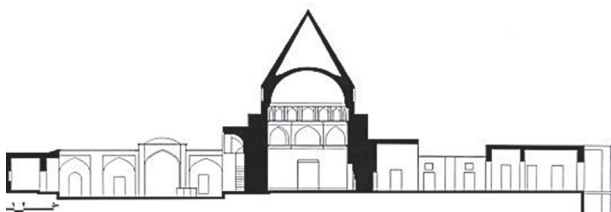
نقشه ۳. برش عمودی ب - ب آرامگاه بابا افضل کاشانی (مأخذ: www.arthut.ir ).
