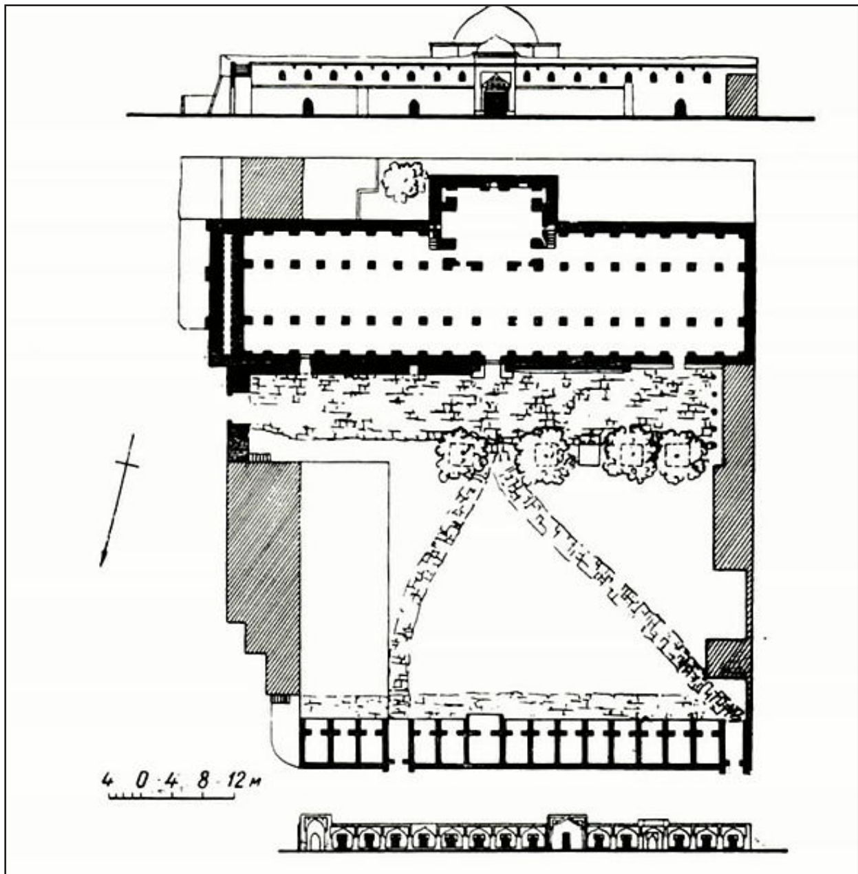
تصویر ۳. نقشه پلان و نماهای مسجد جمعه و مدرسه علوم دینی (مأخذ: مدخل جمعه مسجد، دایرةالمعارف روسی دربند، ۲۰۰۸ م، ص ۱۷۴).
