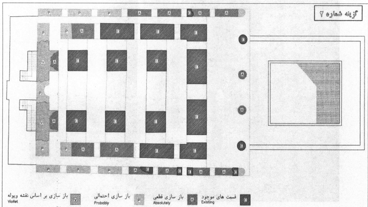
(پلان بازسازی تالار - گزینه شماره ۲ - در این گزینه انتهای تالار بسته است)
