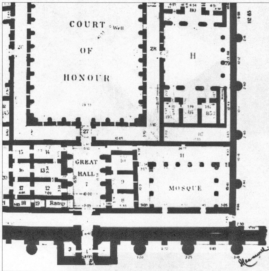
بخشی از پلان مجموعه تاریخی اخیضر، که بناهای مذهبی مجموعه را در خود جای داده است - به پلان مسجد با حیاط رواقدار توجه نمایید
