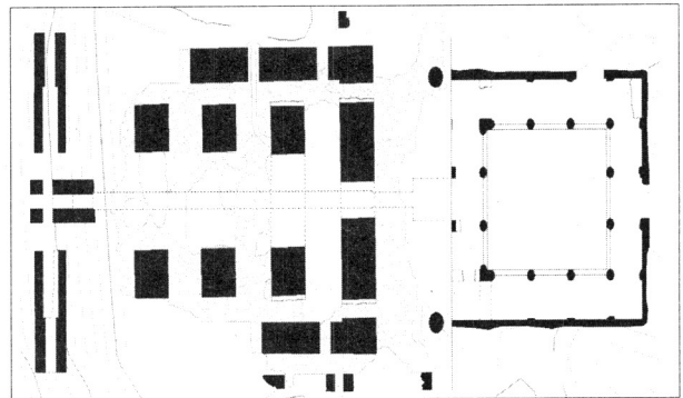
پلان بقایای معماری روی تپه اصلی - محوطه تاریخی تپه میل
