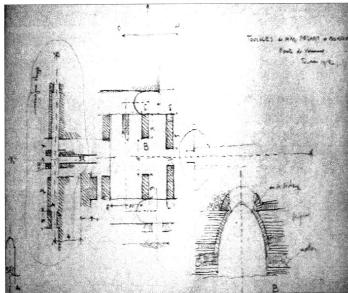
نقشه تهیه شده به وسیله آقای هنری ویوله از تپه میل در ۱۹۱۲
