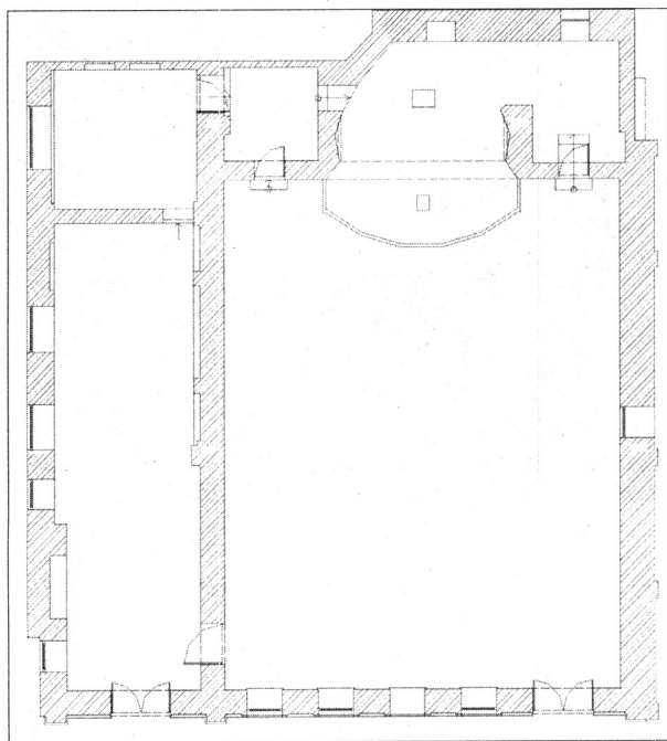
۱۲. دبیرستان کزازی - ساختمان سالن اجتماعات - (پلان)
