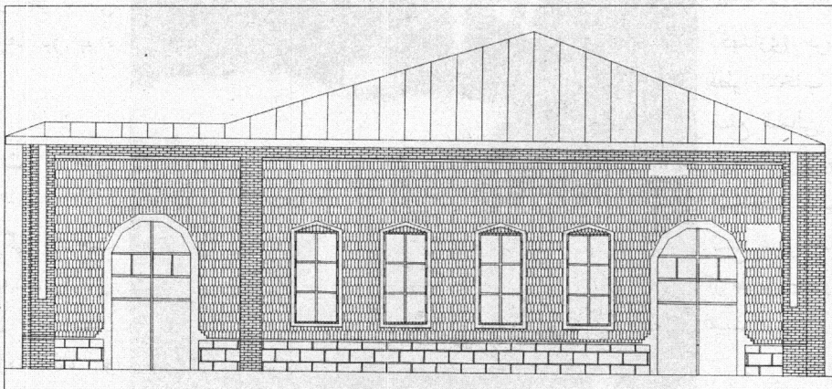
۱۳. دبیرستان کزازی - ساختمان سالن اجتماعات - (نما)
