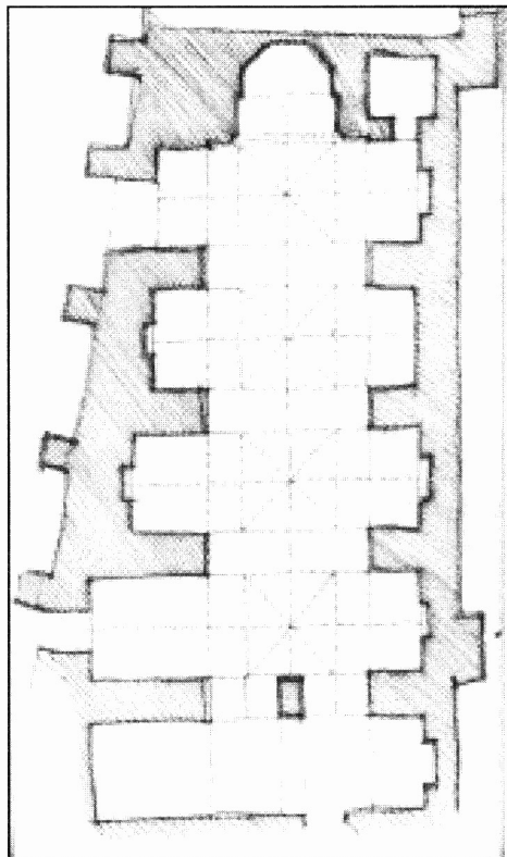
شکل شماره ۲۰-پلان نوع رایج گرمخانه‌های میبد
