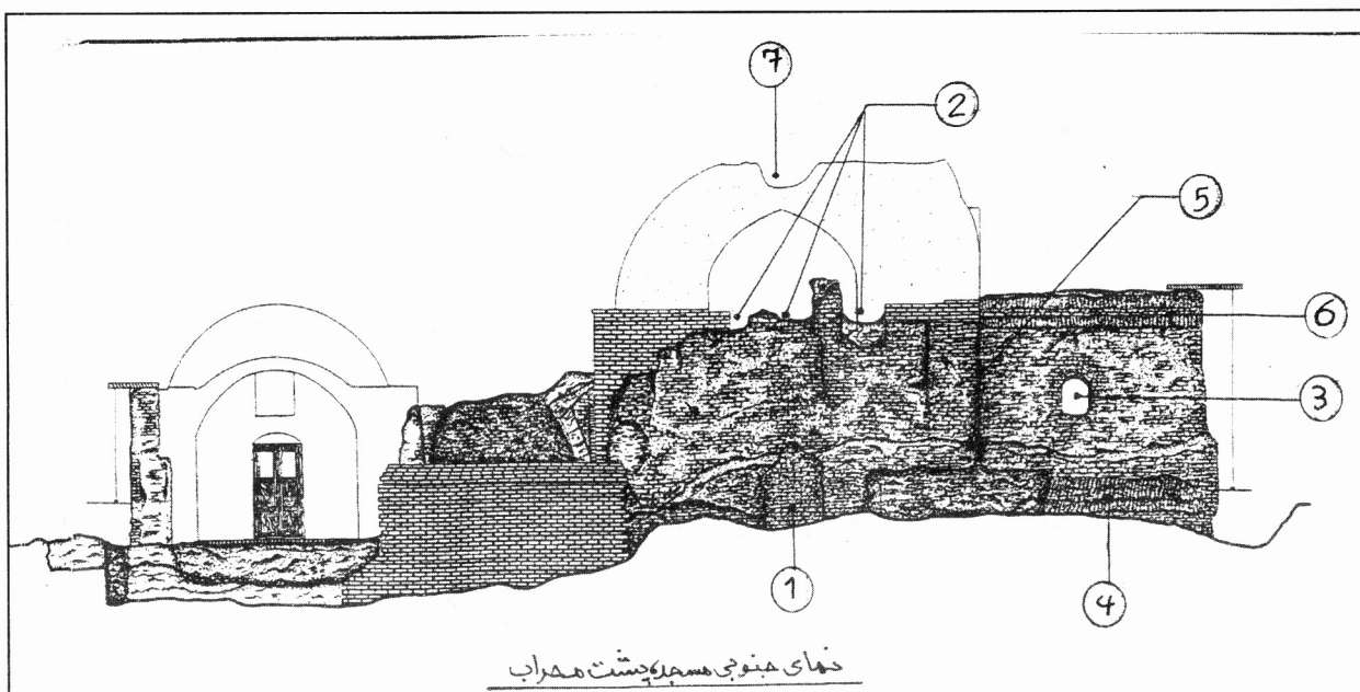
شکل شماره ۵- نمای پشت محراب مسجد
