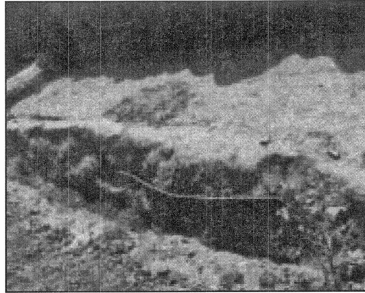
عکس شماره ۲۱ - گرمخانه مسجد ده نو، پس از حفاری و مشخص شدن چرخ غربی
