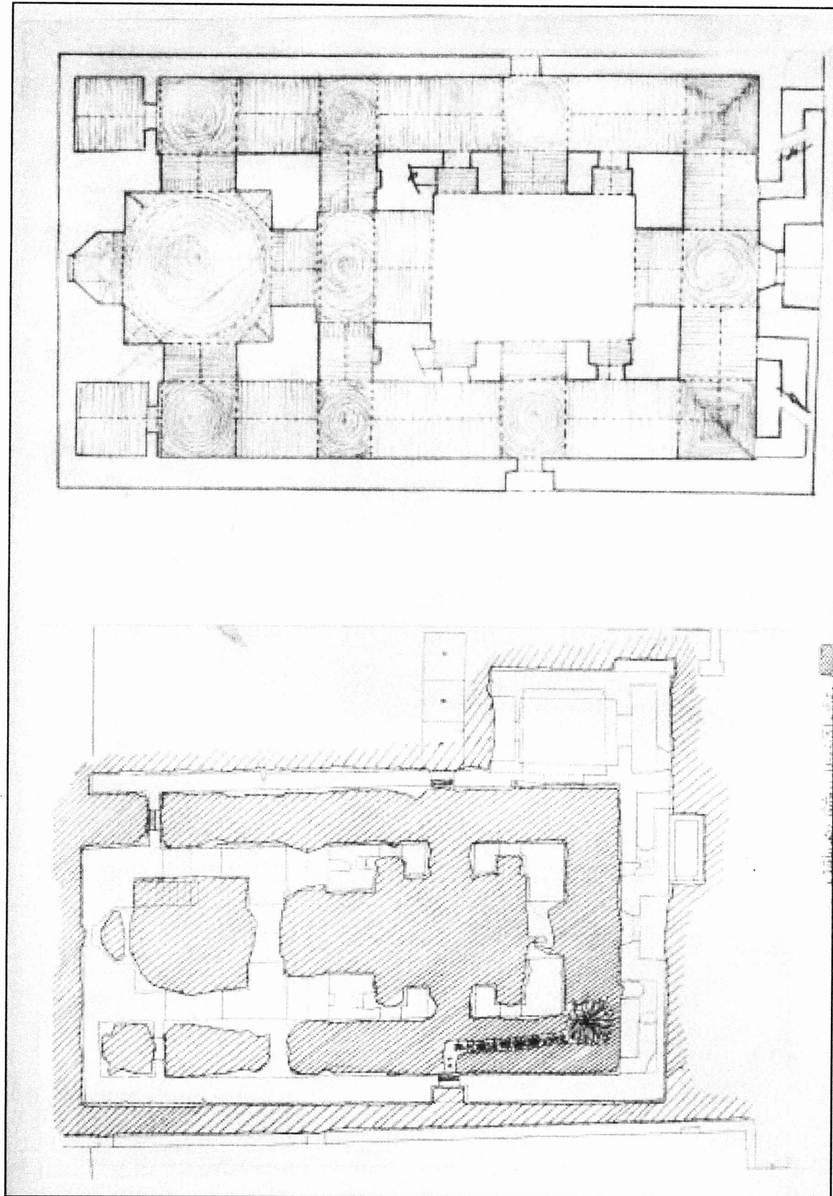
شکل شماره ۳۵ - پلان معکوس از وضعیت موجود سقف‌های از میان رفته مسجد و بازسازی تصویری از وضعیت اولیه آن بر اساس شواهد و مدارک
