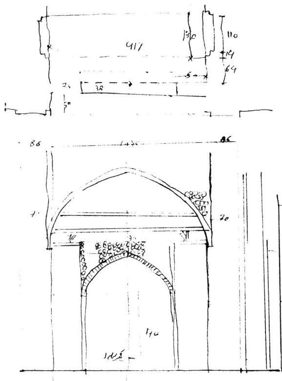
(شکل شماره ۲۷) مسجد جامع ایروان کروکی پلان، نما و مقطع ورودی غربی مقیاس ۱/۶۵، ۷۵/۶/۱۰ شیرازی)
