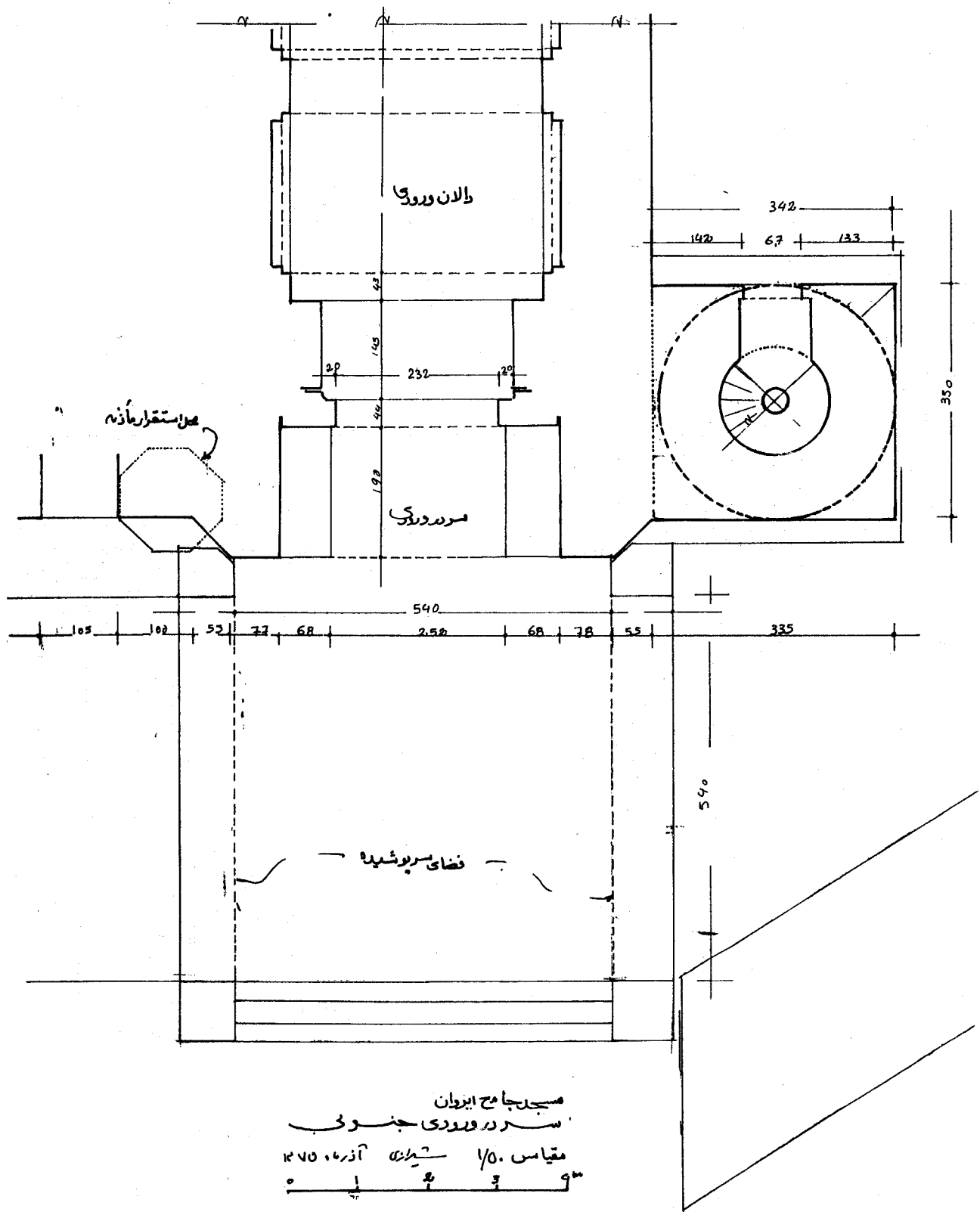
(شکل شماره ۱۵) سردر ورودی جنوبی، مناره، مازنه و پایه‌های سرپوشیده سردر ورودی و دالان ورودی براساس مطالعات و بررسی و کاوشهای سال ۱۳۷۰، توسط نگارنده
