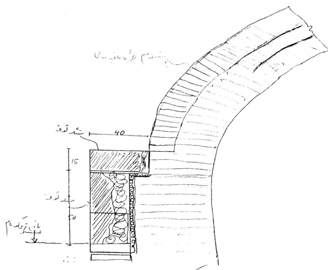
(شکل شماره ۲۵) عایقکاری و آب‌بندی گنبد شبستان شرقی (ایروان)
