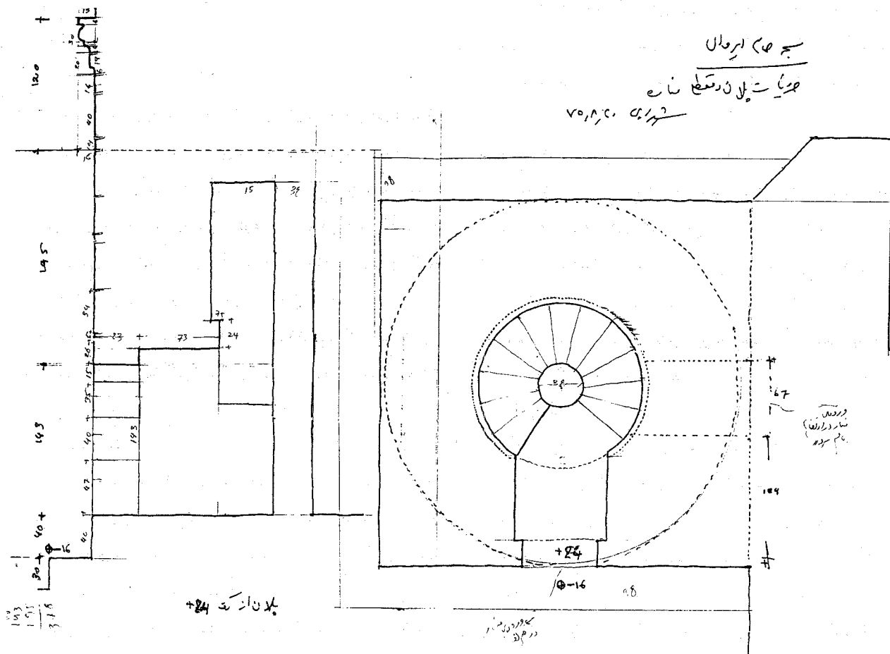
جزئیات پلان و مقطع پایه مناره - شیرازی ۷۵/۸/۲۰
