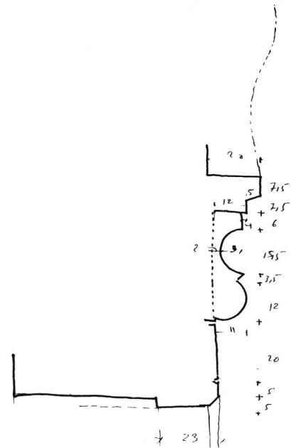
(شکلهای شماره ۲۵ و ۲۶) مسجد جامع ایوان ۷۵/۸/۱۹ جزئیات سنگی زیر آونگ گنبد و روی ساقه مقیاس ۱/۱۵ شیرازی
