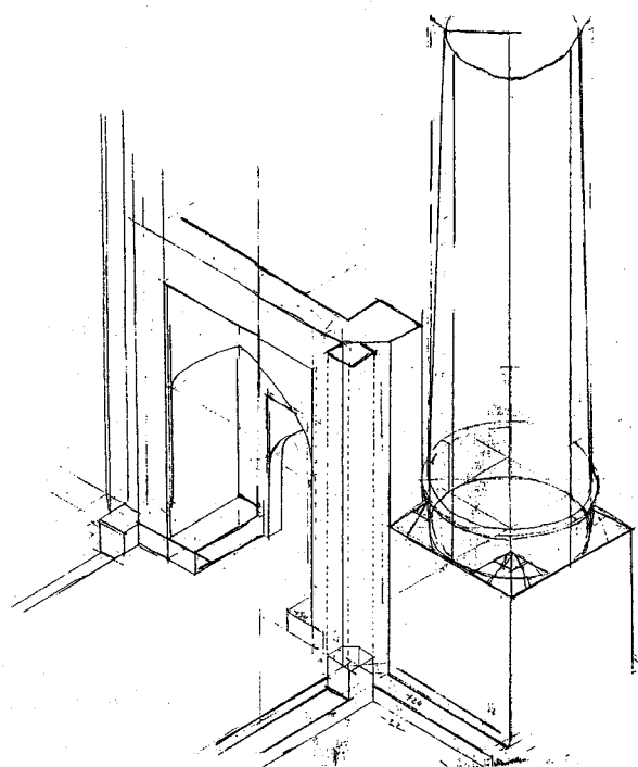
مسجد جامع ایروان (شکل شماره ۱۸) نمای عمومی سردر جنوبی (بازسازی از روی مدارک کاوشها) نگاه از شرق به غرب، مقیاس ۱/۲۵ شیرازی ۷۵/۸/۲۱
