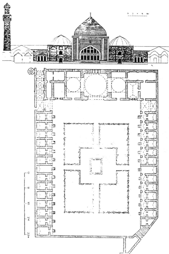
(شکل شماره ۶) مسجد - مدرسه حسین علی خان یا جامع کبود (گوک) نقشه و مقطع عرضی از حیاط و نمای شمالی (گنبدخانه) «ماخذ مقاله مرحوم کونشو»
