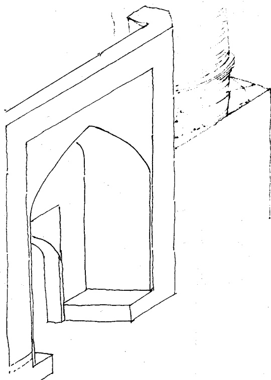
(شکل شماره ۱۹) مسجد جامع ایروان سردر اصلی (جنوبی) نمای عمومی (۷۵/۸/۲۱) مقیاس ۱/۵۰ شیرازی
