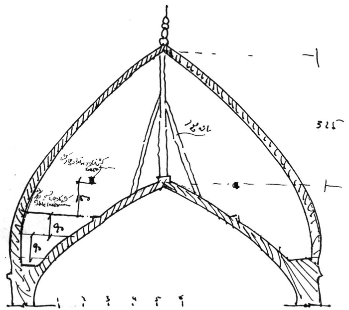
شکل شماره ۲۵) مهارکشی دو پوسته گنبد انجام شده احتمالاً در نیم قرن اخیر مقیاس ۱/۵۵ شیرازی ۷۹/۸/۲۰
