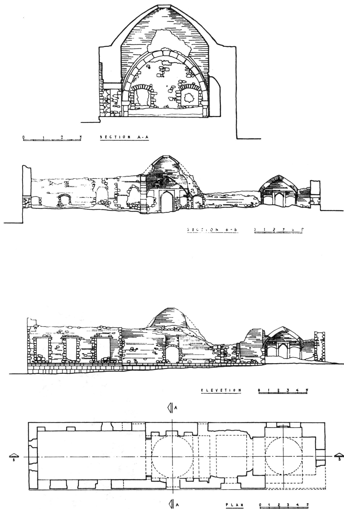
(شکل شماره ۳۵) مسجد روستای آغاراک - مقاطع نما و پلان - «ماخذ مهندس آراکلیان»
