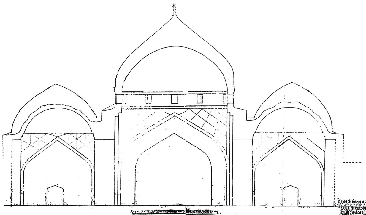
(شکل شماره ۱۲) مقطع شرقی غربی هسته جنوبی مسجد جامع ایروان (ماخذ اداره کل حفاظت آثار تاریخی ارمنستان)
