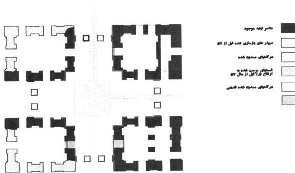
طبقه همکف چشمه عمارت بهمن - زمستان ۱۳۰۳ م: ۱:۱۰۰
