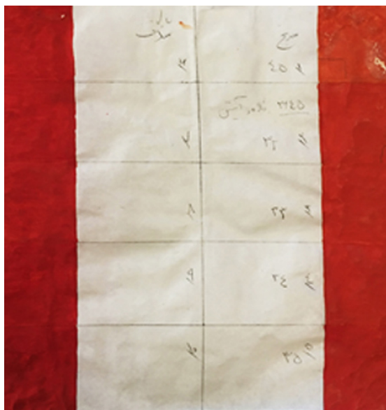
شکل ۴. نمونه جداول رنگ های آماده سازی شده بر پایه سرنج - سنگرف.
