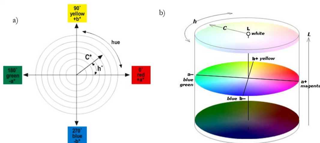
شکل ۲. (a) زاویه فام و خلوص در فضای رنگ CIELCH
