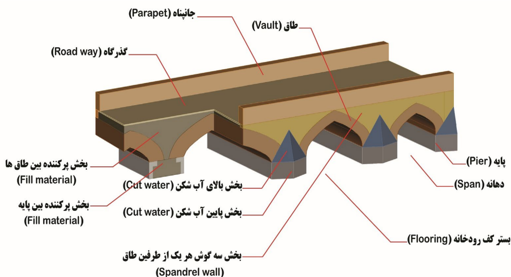
شکل ۵. اجزای معماری سازنده پل
