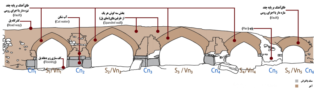
شکل ۷. نمای شمالی و عناصر تشکیل دهنده پل در این نما
