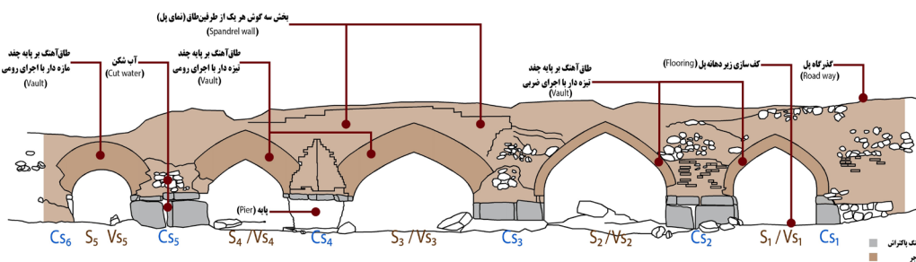
شکل ۸. نمای جنوبی و عناصر تشکیل دهنده پل در این نما
