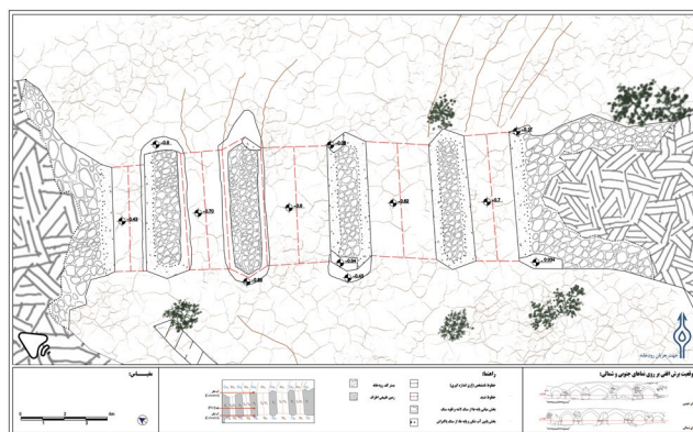
شکل ۶. پلان پل تاریخی ایزدخواست
