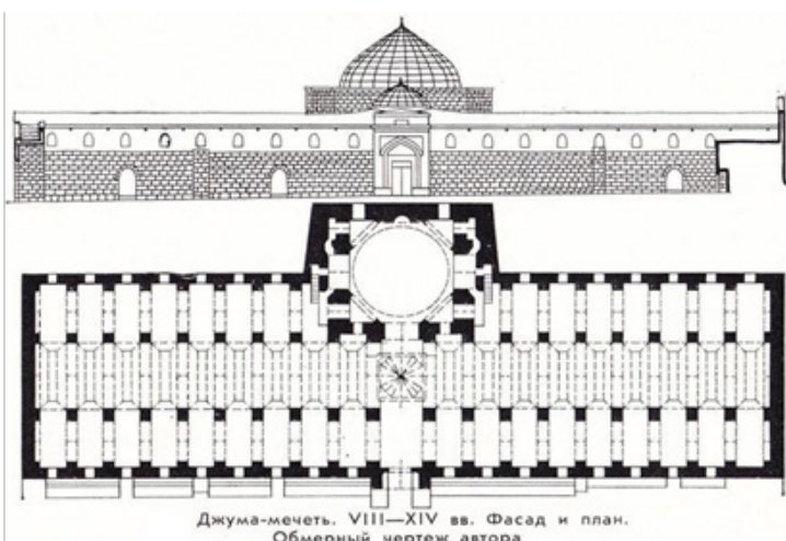
شکل ۱. پلان مسجد جمعه و مدرسه علوم دینی، (ماخذ: Quba-Xaomaz, 2008, 174)
