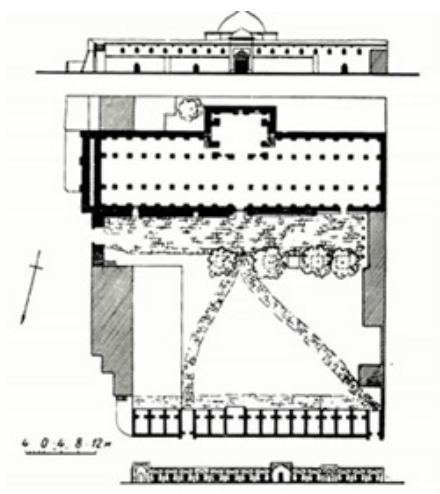
شکل ۱. پلان مسجد جمعه و مدرسه علوم دینی، (ماخذ: Quba-Xaomaz, 2008, 174)
