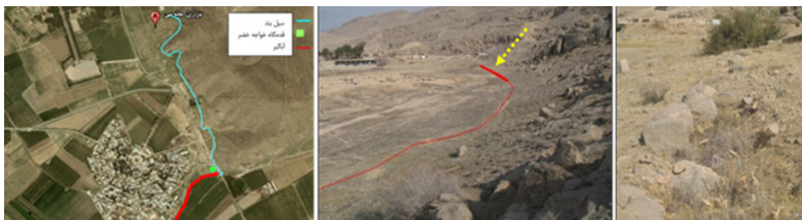
شکل ۴: تدبیر هخامنشیان به منظور جلوگیری از نفوذ سیلاب‌های کوهستان به درون شهر در قسمت مشخص شده پی‌سازی سیل بند قابل مشاهده است. موقعیت آبگیر شهرک زراعی و سیل بندهای شهر پارسه (نگارندگان، ۱۳۹۵)
