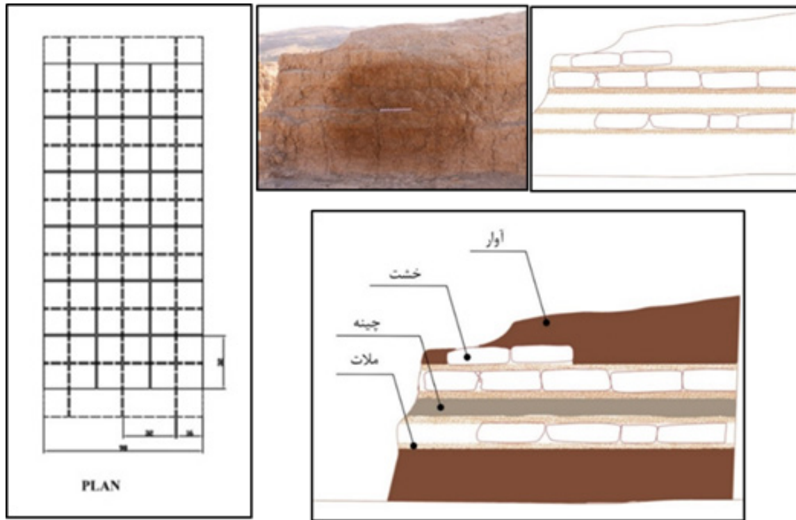
شکل ۹: نحوه چینش و هشت‌گیر کردن خشت‌ها در دیوار
